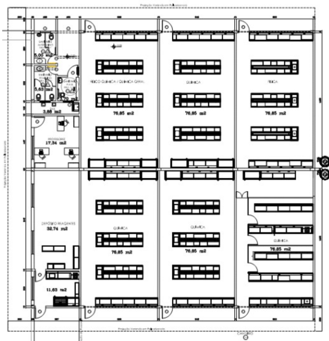
Figura 6 - Planta Baixa dos Laboratórios de Química e Física.
